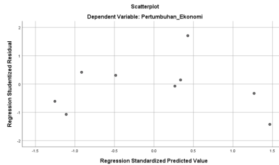
Gambar 1. Uji Heterokedastisitas
